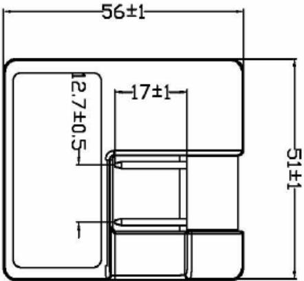
AC PIN 折叠180°
